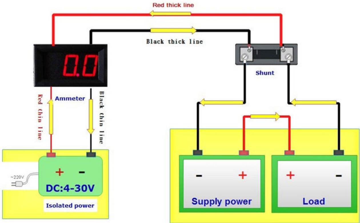
Схема подключения прибора при питании от измеряемой схемы:
